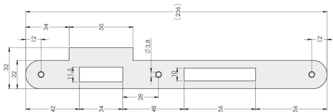
PRIHVATNIK ZA MEHANIČKE BRAVE TIP B
