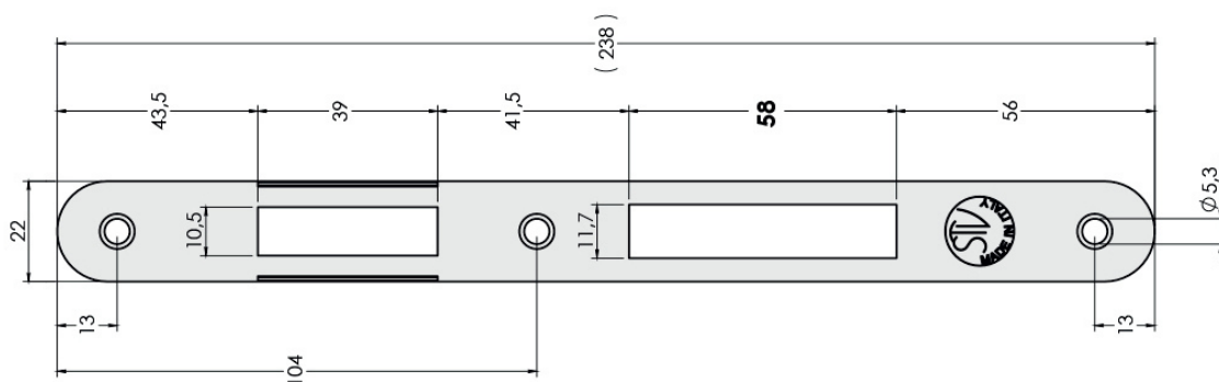
PRIHVATNIK ZA MEHANIČKE BRAVE TIP A2
